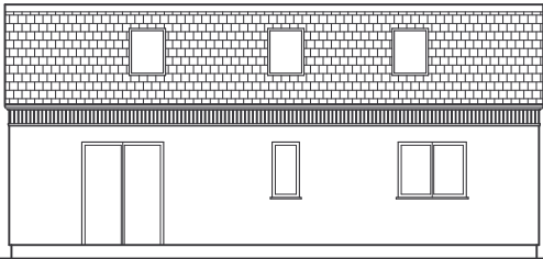
ELEWACJA TYLNA
