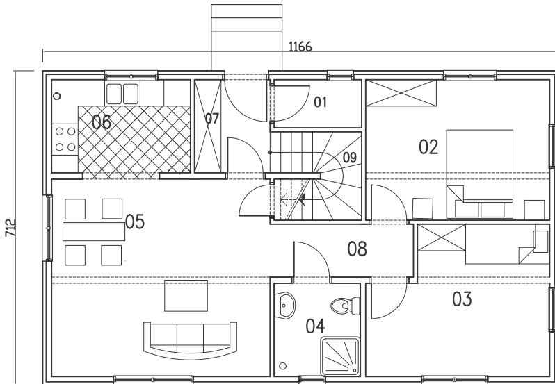
RZUT PARTERU
